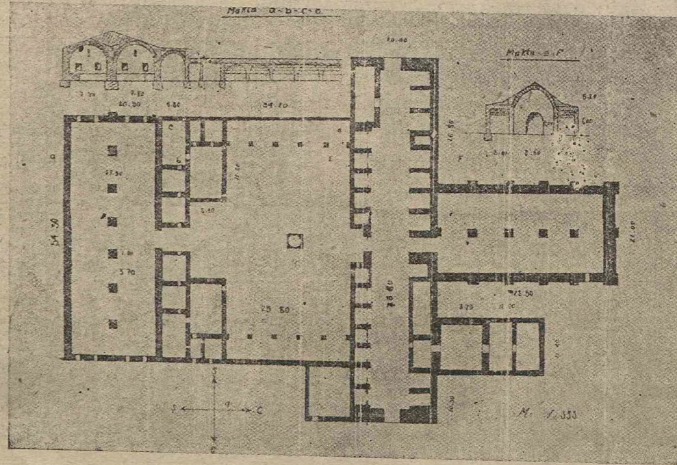
( Resim 2 ) Ulukışla hanının plânı
