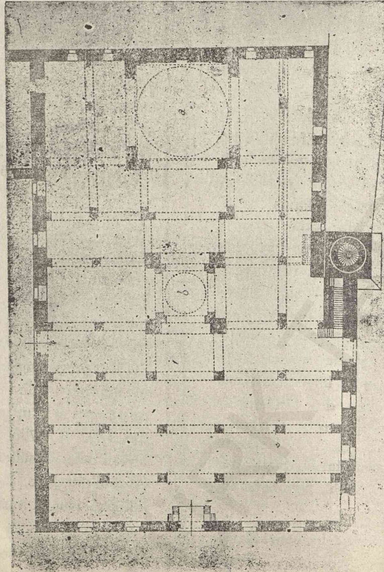
Raşit Efendi Kütüphanesi ve Ulucami plânı [12]
