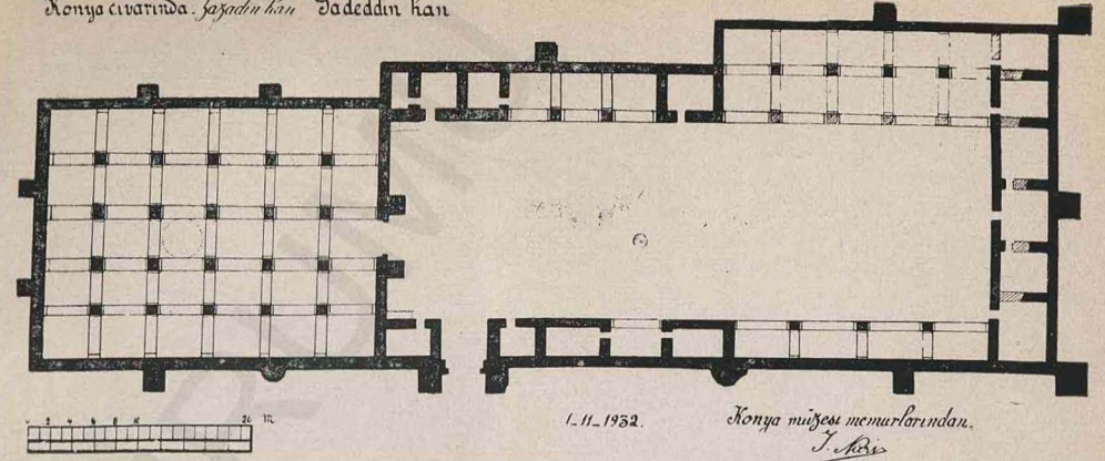
Zazadın (Sadeddin) Hanının Plânı
