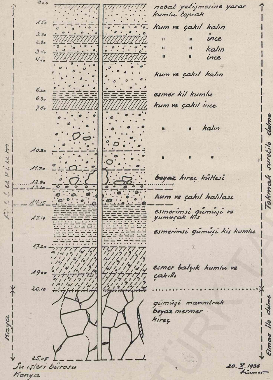
Altınapada yapılan sondajın maktai (Tabakalar)
