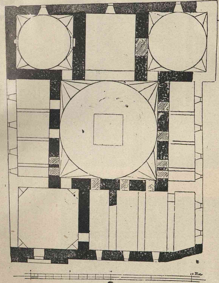
Konya'da Büyük Karatay Medresesi plânı
