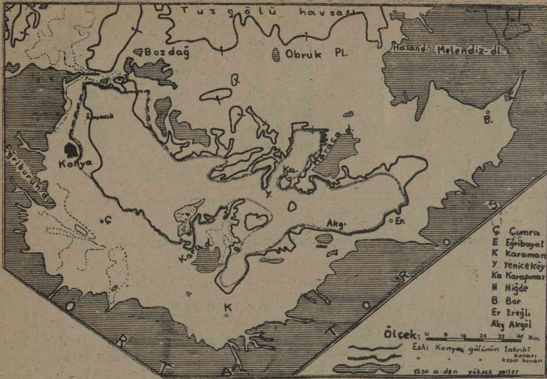
Buzul devrinde Konya - Ereğli gölü.
